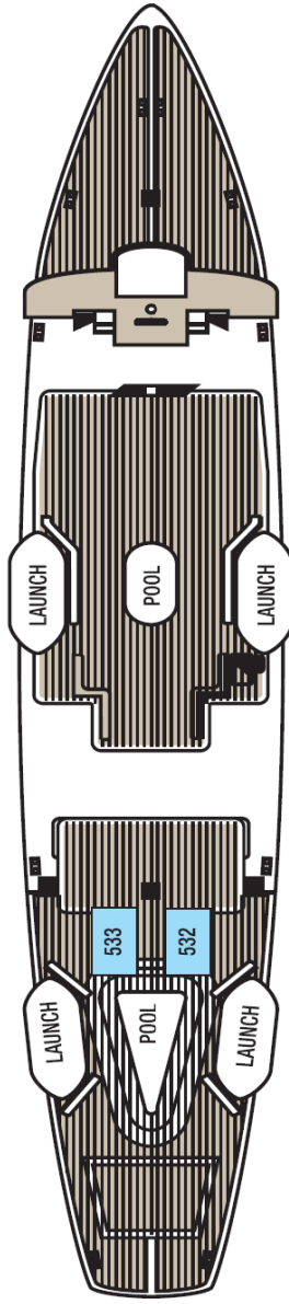
Sun
